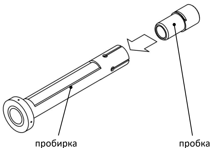
Рисунок 12. Сборка датчика по ISO. Этап 1
