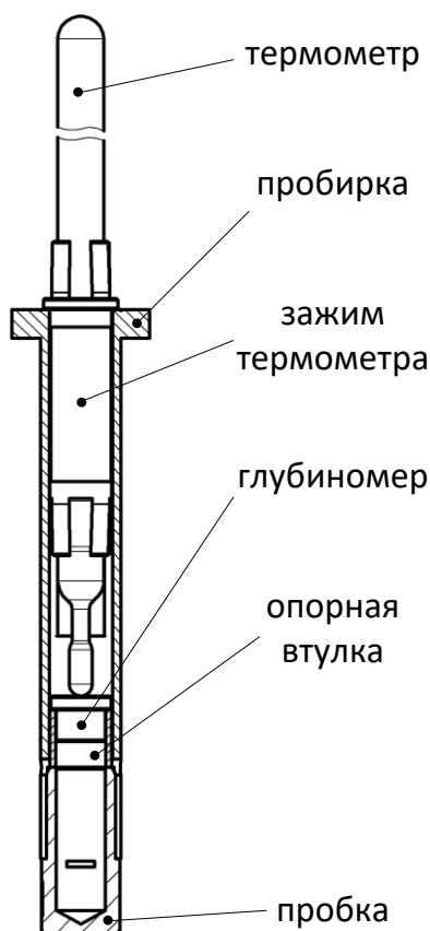
Рисунок 7. Сборка датчика по ГОСТ. Этап 2
