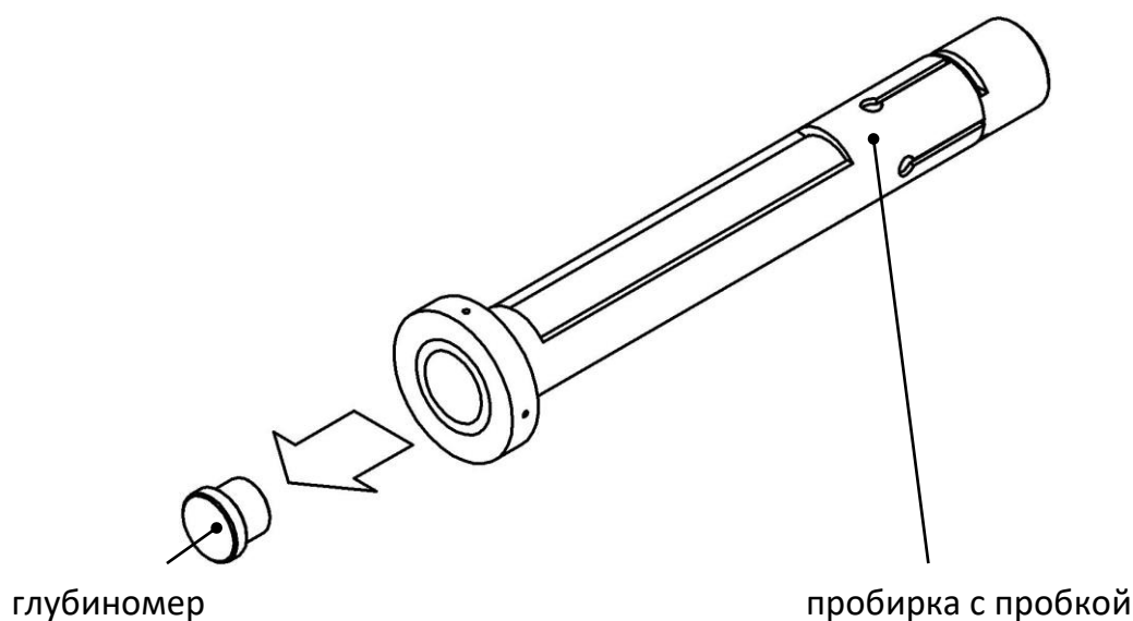
Рисунок 14. Сборка датчика по ISO. Этап 3
