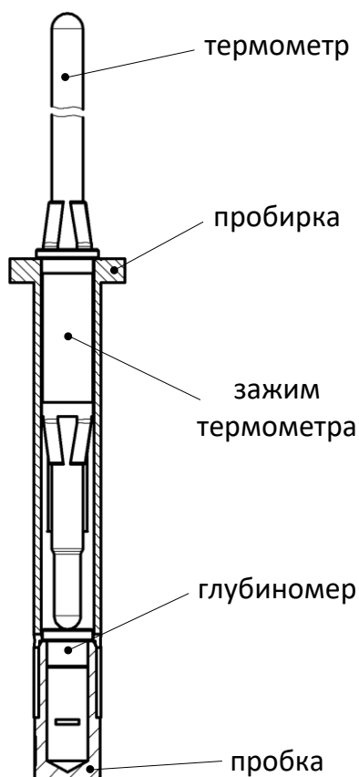
Рисунок 13. Сборка датчика по ISO. Этап 2
