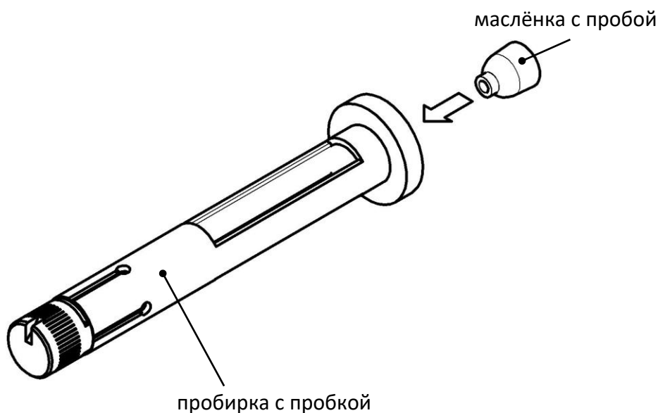
Рисунок 16. Сборка датчика по ISO. Этап 4
