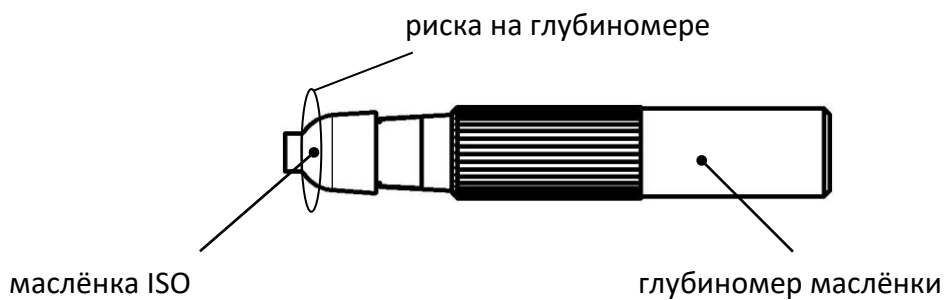
Рисунок 11. Проверка геометрии маслѐнки ISO
