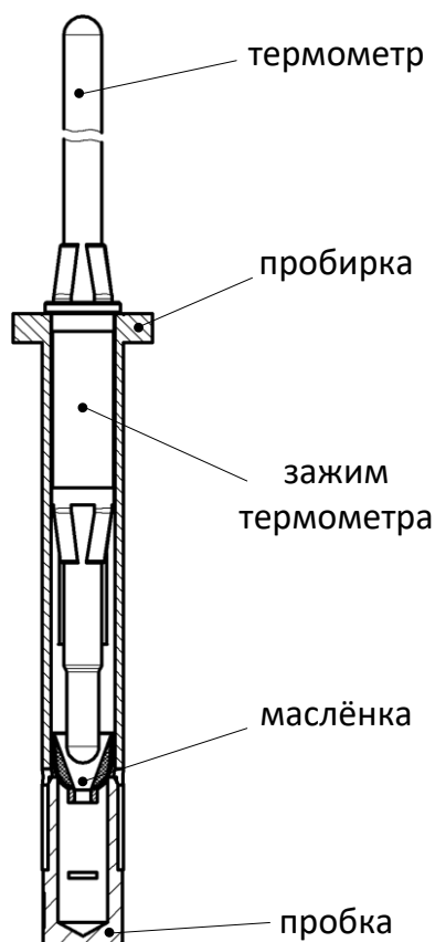
Рисунок 17. Датчик по ISO с установленным термометром
