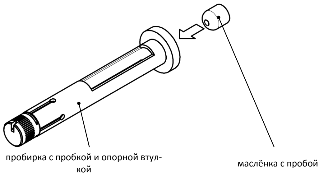
Рисунок 8. Сборка датчика по ГОСТ. Этап 3
