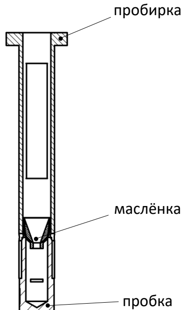
Рисунок 18. Датчик по ISO без установки термометра
