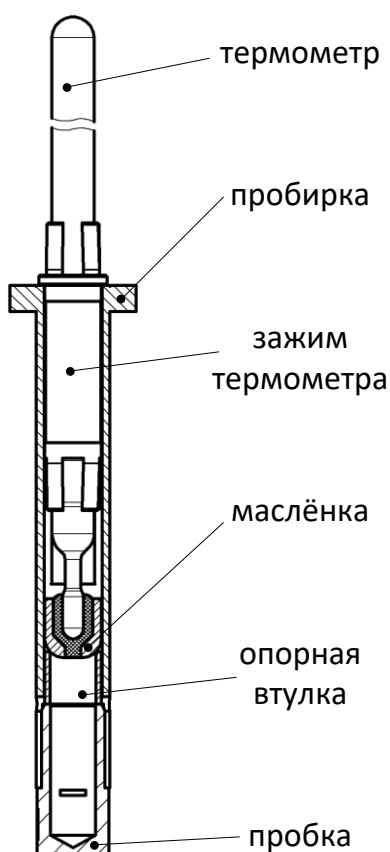
Рисунок 9. Датчик по ГОСТ с установленным термометром
