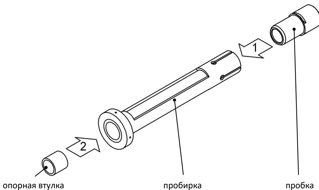
Рисунок 6. Сборка датчика по ГОСТ. Этап 1
