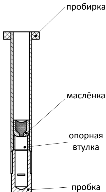
Рисунок 10. Датчик по ГОСТ без установки термометра
