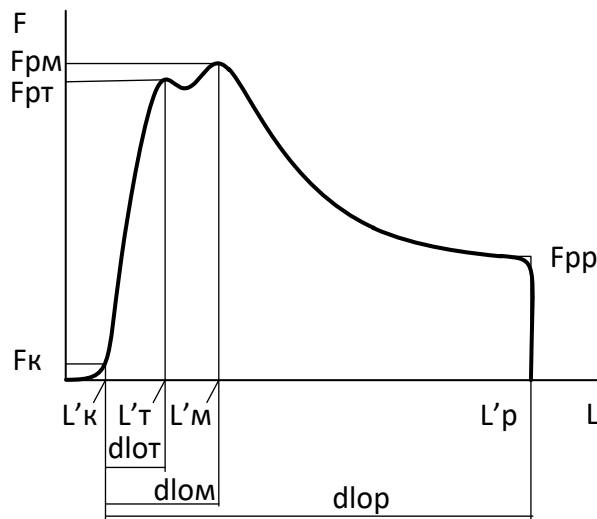
Fpт – усилие текучести (условная текучесть не определяется); Fpm – усилие прочности (максимальное усилие); Fpp – усилие разрыва; dлот – удлинение, соответствующее усилию текучести; dlom – удлинение, соответствующее усилию прочности; dlор – удлинение, при котором был зафиксирован разрыв; L'к – положение каретки, при котором зафиксировано касание образца; L'т – положение каретки, соответствующее усилию текучести; L'м – положение каретки, соответствующее усилию прочности; L'р – положение каретки, при котором зафиксирован разрыв образца.
