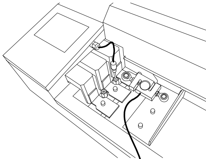
Рисунок 30 – Установка образцового динамометра
