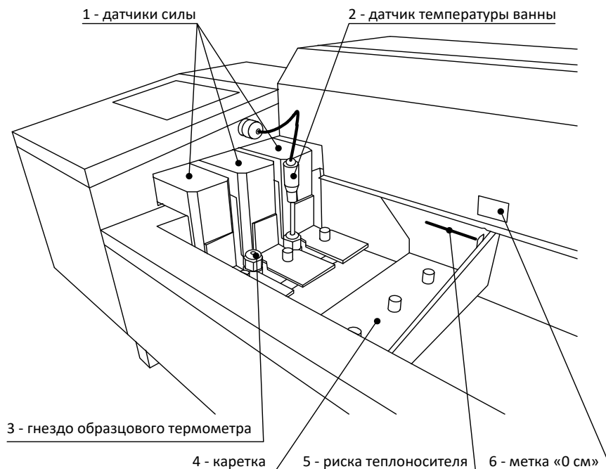
Рисунок 4 – Система нагружения
